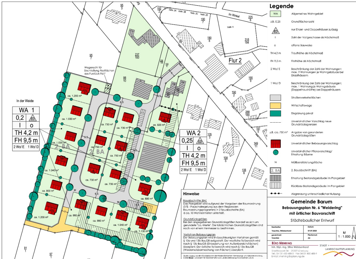
Abb.2: Städtebaulicher Entwurf zum Bebauungsplan Nr. 6 „Weidering“ mit ÖBV der Gemeinde Barum (ohne Maßstab). Quelle: Büro Mehring (2023).
